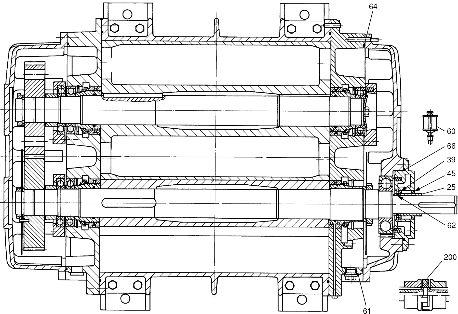
Abb. / Fig. 3 RUVAC RA 9001
