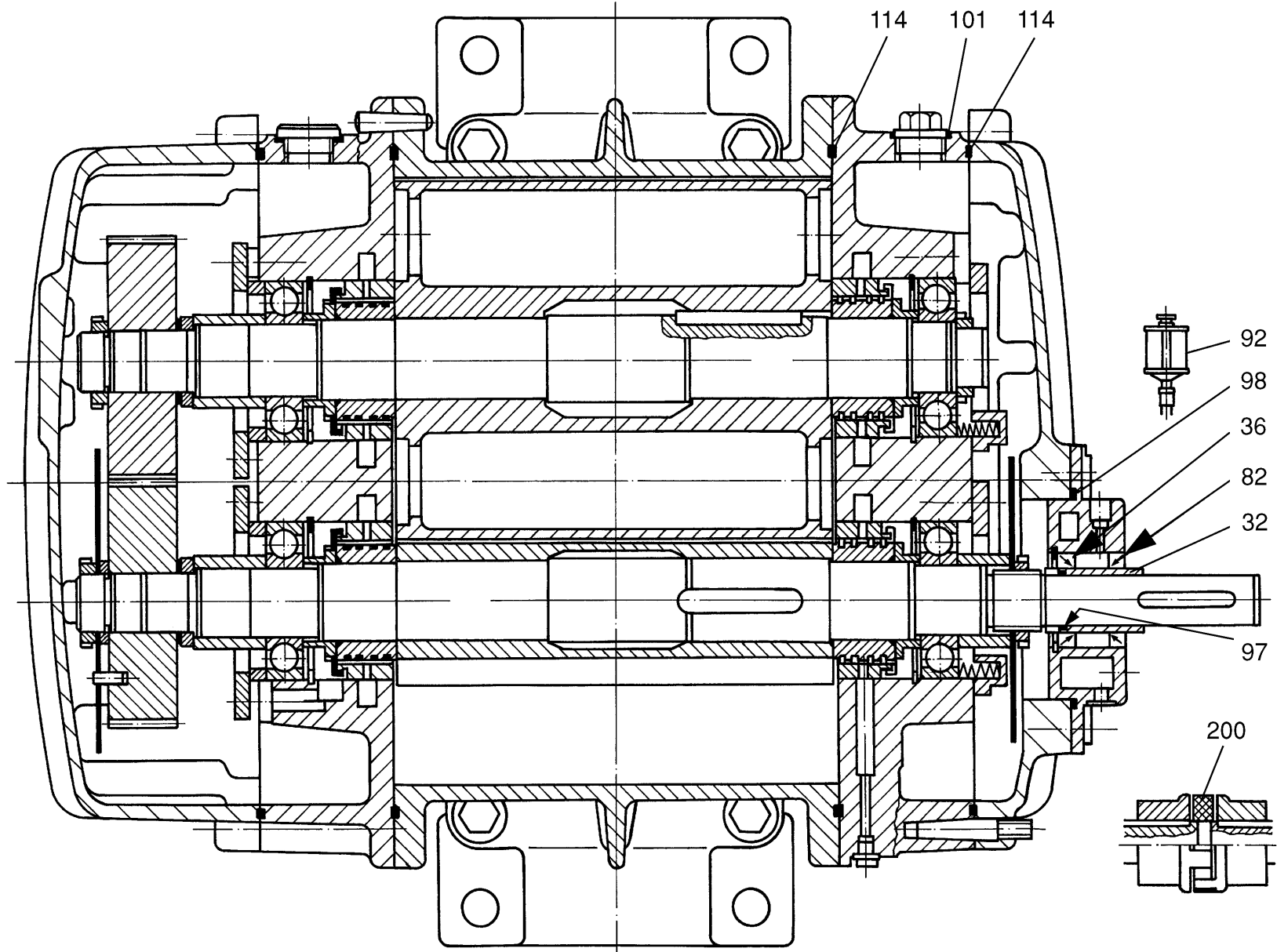
Abb. / Fig. 1 RUVAC RA 3001
