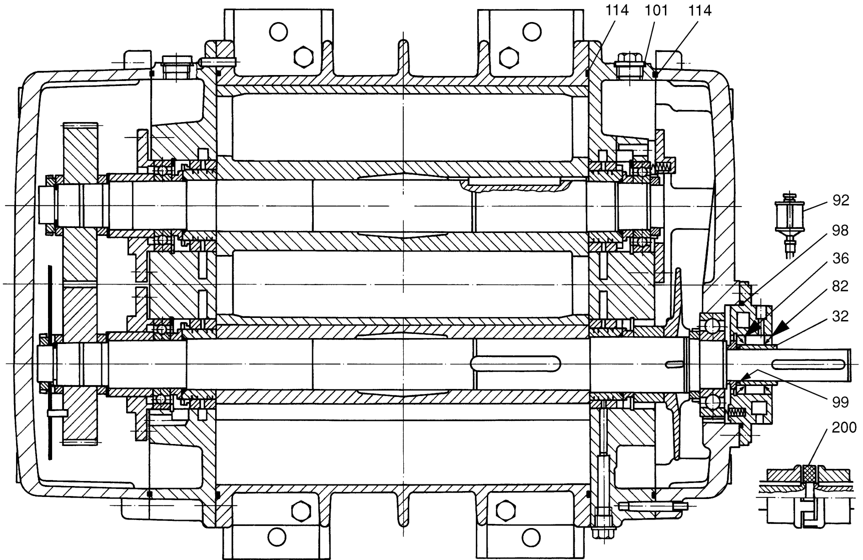
Abb. / Fig. 2 RUVAC RA 5001, RA 7001
