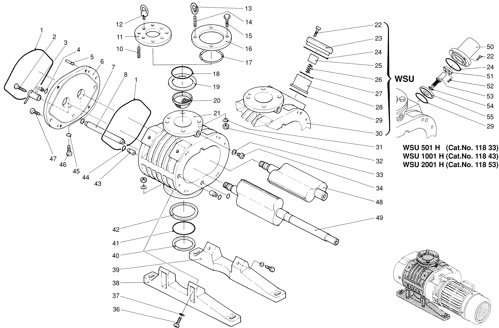
Abb./Fig. 2 RUVAC WS/WSU
