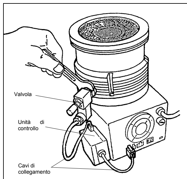
Installazione
